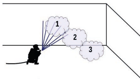
Imagen 83. Enfriamiento de gases tradicional con pulsaciones cortas de corto alcance
