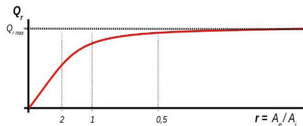
Imagen 109. Variación del caudal efectivo ( Q_r ) y la relación ( r ) entre la salida de gases ( A_e ) y la entrada ( A_i ). Una entrada dos veces el tamaño de la salida da resultados más que suficientes
