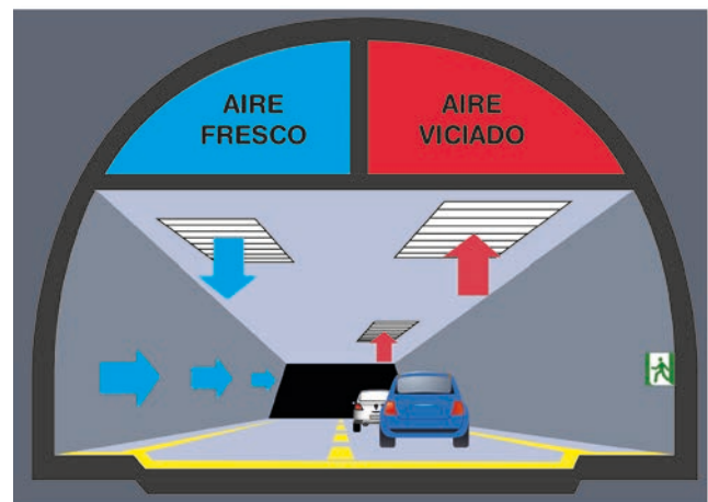
Imagen 5. Ventilación transversal
