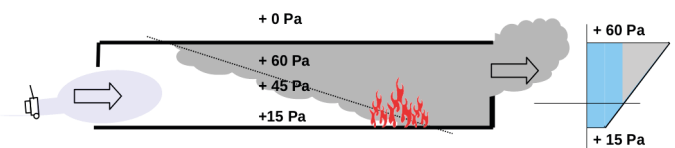
Imagen 69. Distribución de diferenciales de presión en un recinto de incendio sometido a ventilación VPP
