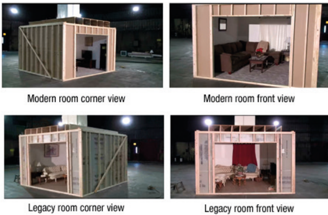
Imagen 5. Detalle de la configuración del experimento de comparación de combustible moderno y tradicional
