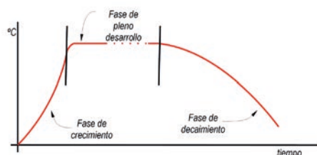
Imagen 8. Curva de evolución de la temperatura mostrando las fases de desarrollo de un incendio de interior
