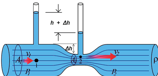
Imagen 16. Efecto Venturi
