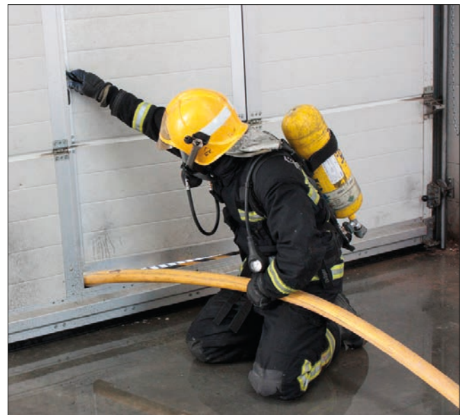
Imagen 153. Puerta entornada a la anchura de paso de la manguera
