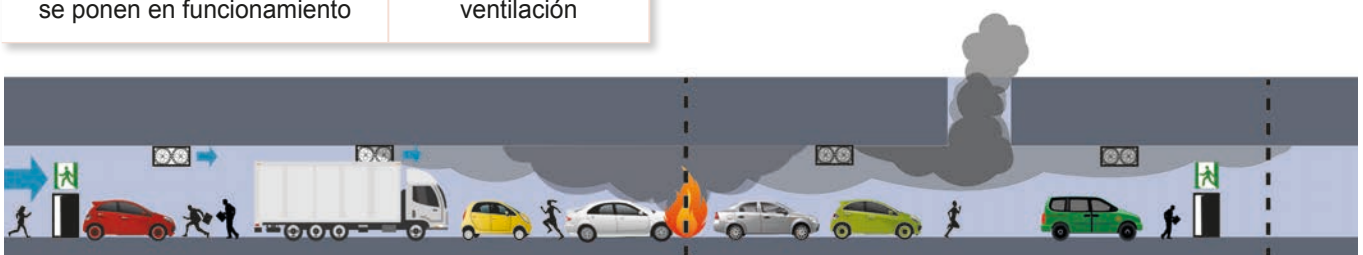
Imagen 3. Túnel de ventilación longitudinal con extracción masiva de humo
