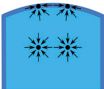
Imagen 3. Tensión superficial
