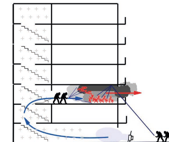
Imagen 186: Ataque combinado (ataque exterior ofensivo + enfriamiento de gases + APP)
