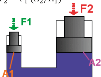
Imagen 9. Prensa hidráulica
