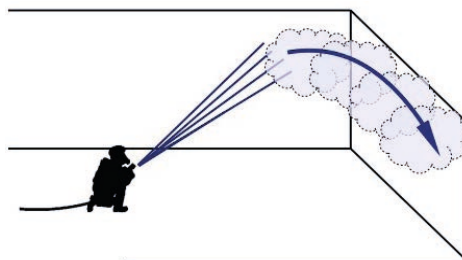
Imagen 84. Enfriamiento de gases con pulsaciones más largas y de largo alcance
