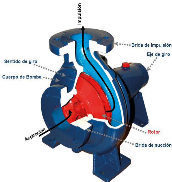
Imagen 18. Bomba centrífuga
