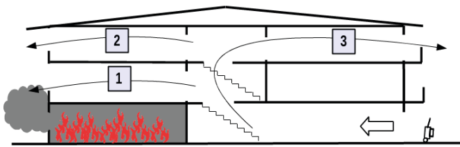
Imagen 141. Ventilación secuencial en una operación de ventilación defensiva para limpiar de humo todas las estancias de bloque de viviendas
