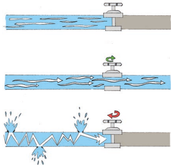
Imagen 17. Golpe de ariete
